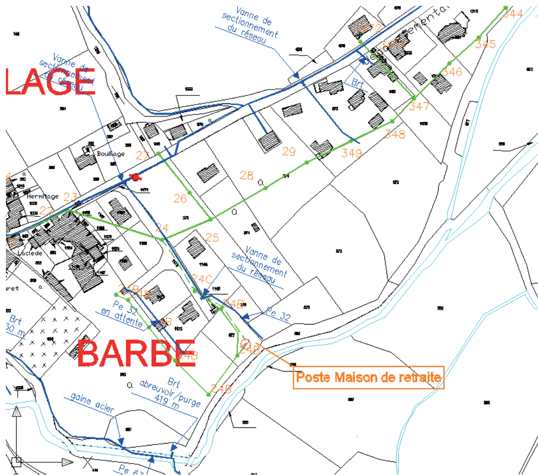
Extrait des réseaux d'alimentation en eau potable (AEP) et d'assainissement sur le secteur Barbe
